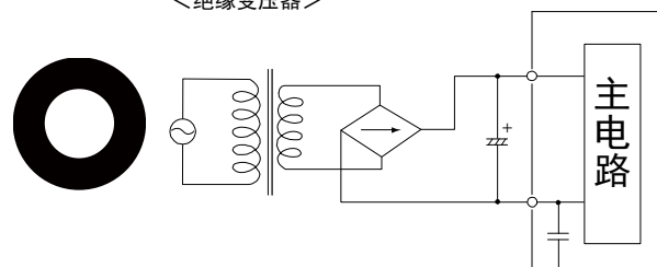
<绝缘变压器>
